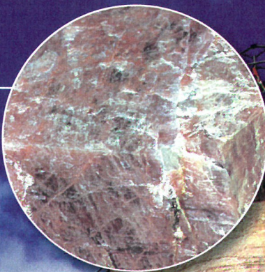
Feldspar
