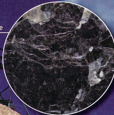
Biotite
